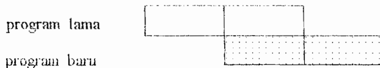
Gambar 4.4. Metode Paralel
