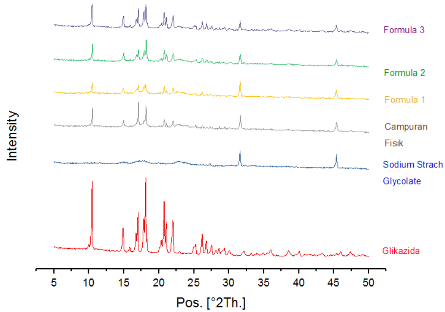
Gambar 4. Difraktogram XRD Gliklazida, SSG, Campuran Fisik, dan Dispersi Padat
