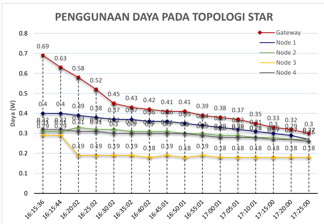
Gambar 4.1 Grafik penggunaan daya pada jaringan sensor nirkabel dengan topologi star
