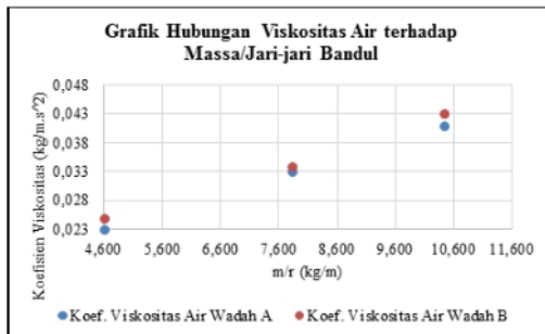
Gambar 4 Grafik hubungan viskositas air terhadap massa/jari-jari bandul
