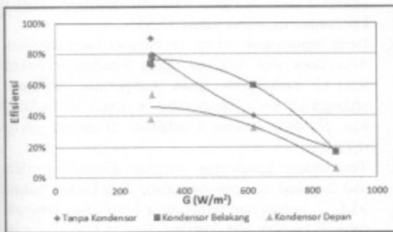
Gambar 7. Efisiensi yang dihasilkan ketiga konfigurasi alat
