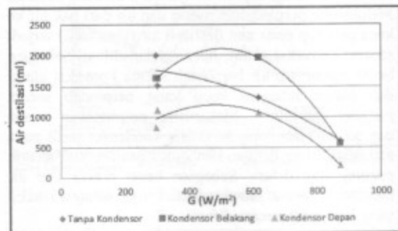
Gambar 6. Air destilasi yang dihasilkan ketiga konfigurasi alat
