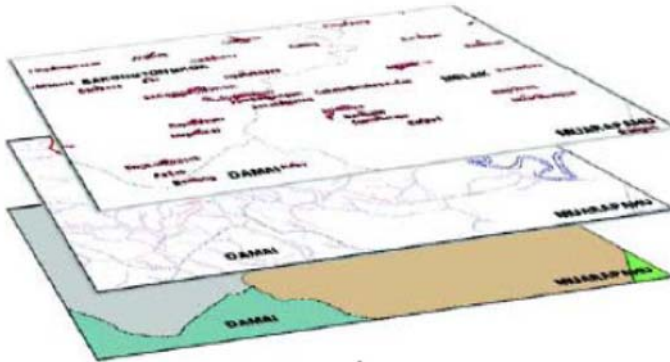
Gambar 1. Konsep Layer
