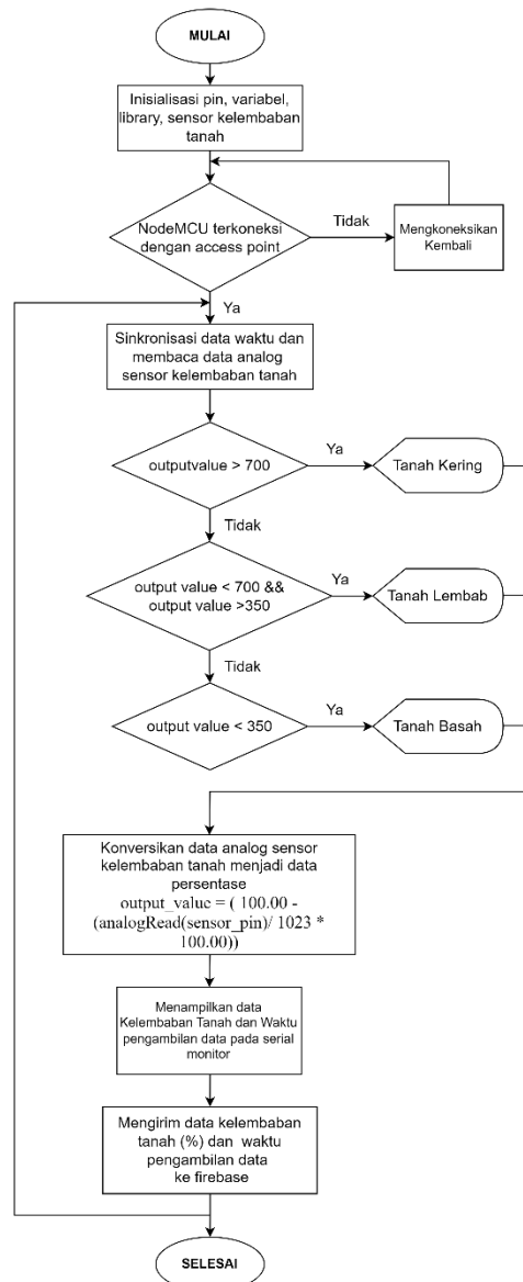
Gambar 2. Diagram alir NodeMCU
