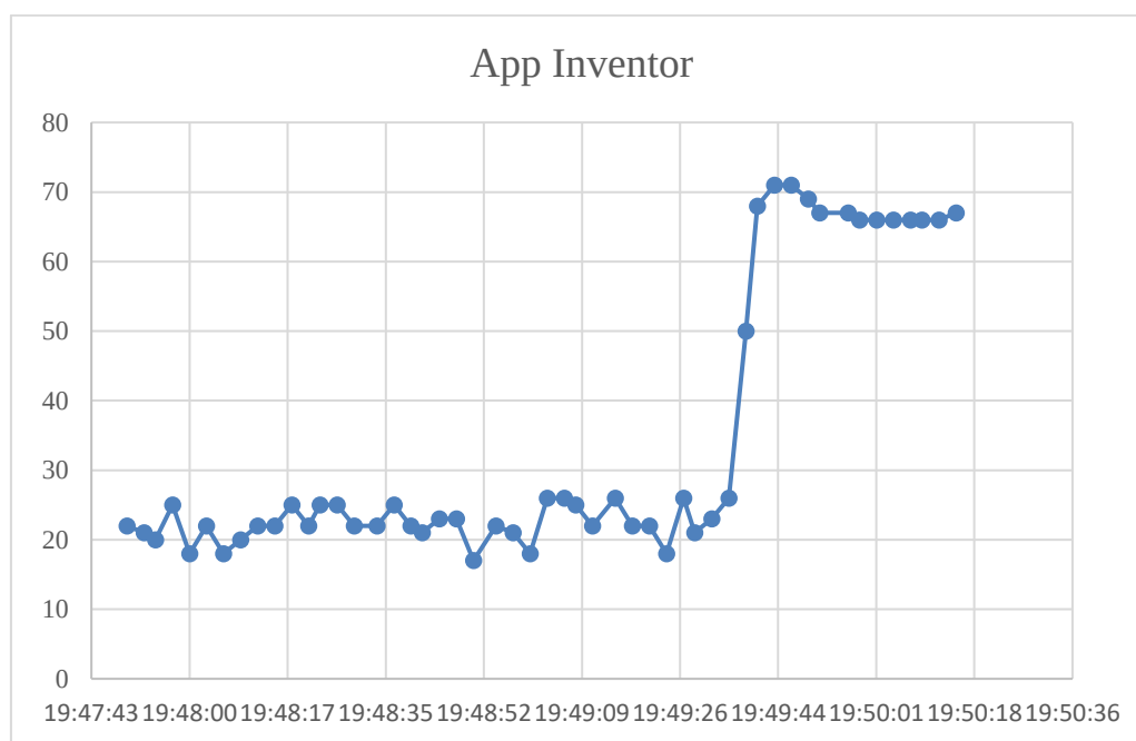
Gambar 7. Grafik Kebocoran Sensor 1 di dalam tanah
