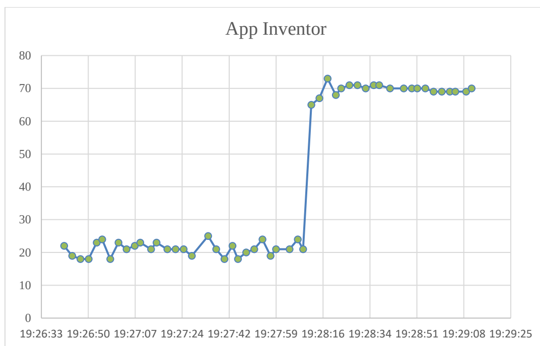
Gambar 6. Grafik Kebocoran Sensor 1 di permukaan
