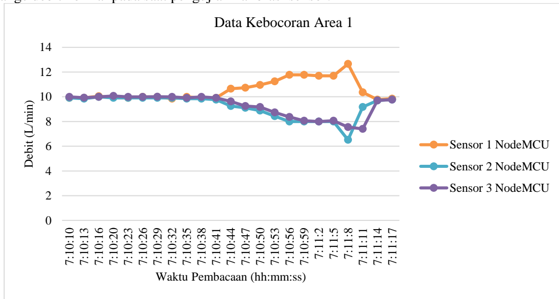
Gambar 7. Grafik kebocoran area 1
