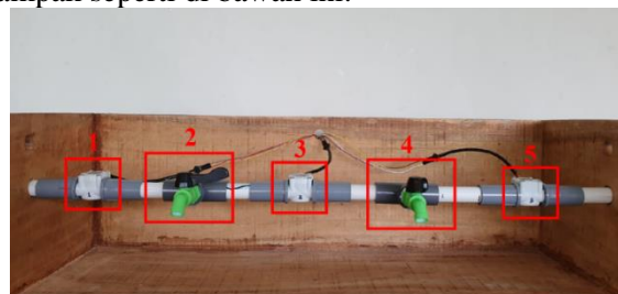
Gambar 1. Bagian dalam boks kayu
