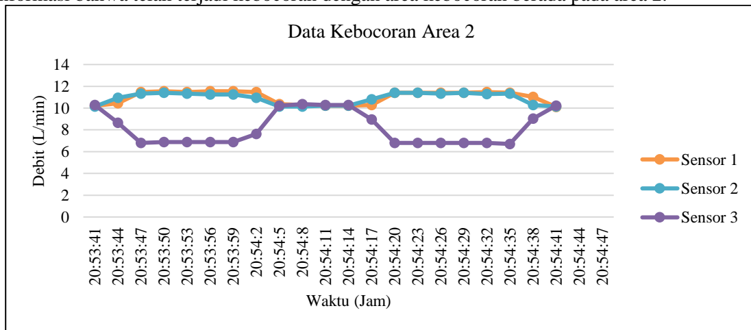
Gambar 9. Grafik terjadinya kebocoran area 2
