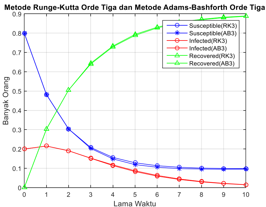
GAMBAR 4. Perbandingan Solusi Metode Runge-Kutta Orde Tiga (RK3) dan Metode Adams-Bashforth Orde Tiga (AB3)
