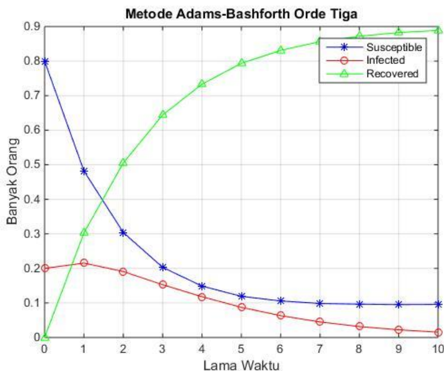
GAMBAR 3. Grafik Solusi Model Epidemiologi SIR dengan Vaksinasi Konstan Menggunakan Metode Adams-Bashforth Orde Tiga
