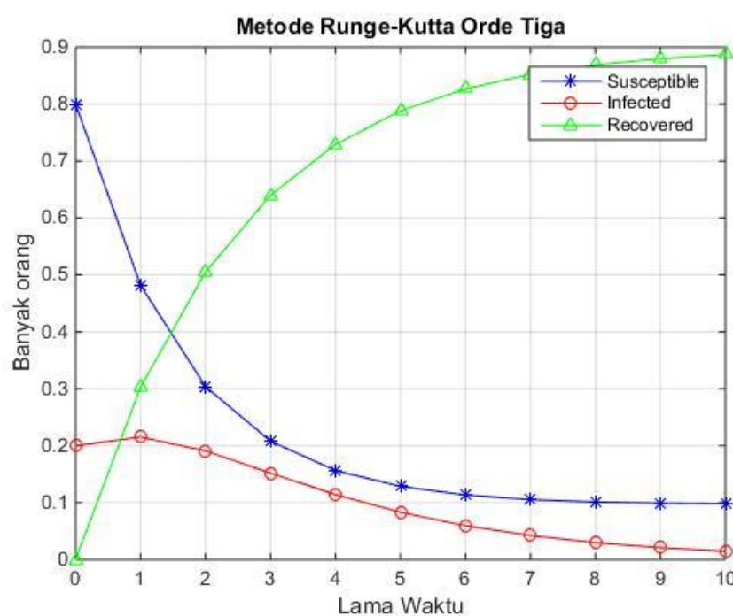
GAMBAR 2. Grafik Solusi Model Epidemiologi SIR dengan Vaksinasi Konstan Menggunakan Metode Runge-Kutta Orde Tiga
