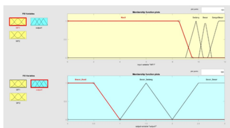
Gambar 6. fungsi keanggotaan input dan output area 1
