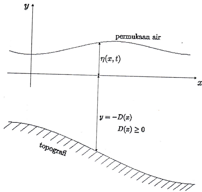
Gambar 1: Aliran air dangkal satu dimensi.
