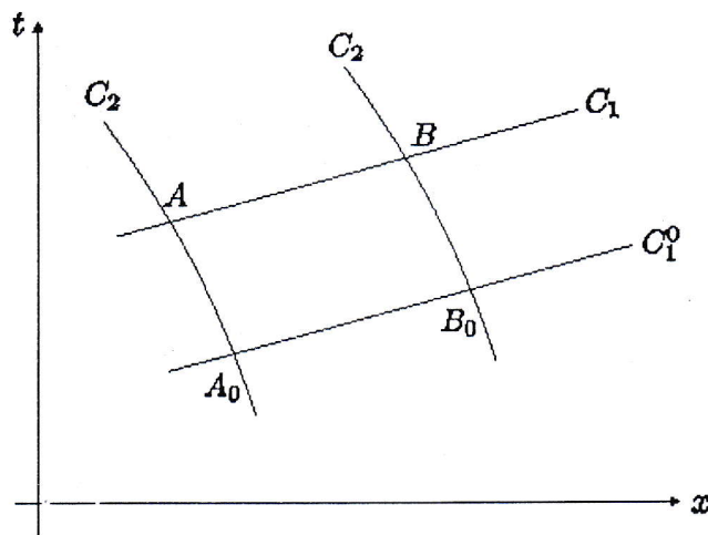
Gambar 2: Suatu daerah dalam bidang- x, t yang memuat karakteristik garis lurus.
