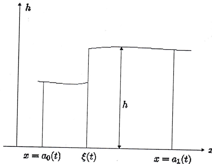
Gambar 3: Suatu keadaan diskontinuitas.
