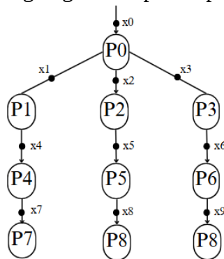
Gambar 2. Petri Net Sistem Pelayanan di SPBU Pertamina Giwangan Yogyakarta
