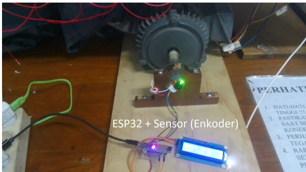
Gambar 5. Pemasangan perangkat ESP32 + Sensor Enkoder untuk memonitor kondisi motor induksi dari jarak jauh dan menampilkan datanya di LCD16x2
