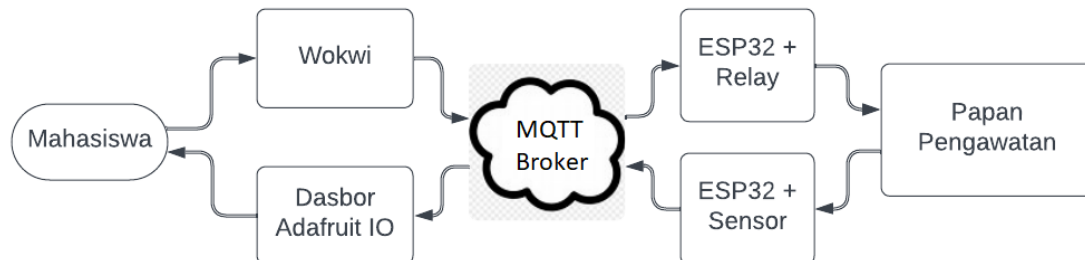
Gambar 2. Konsep pengembangan laboratorium jarak jauh
