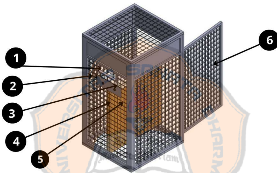
Gambar 3.1 Desain Mesin Trash2Cash
