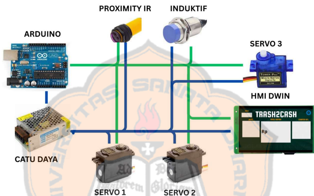
Gambar 3. 5 Rangkaian Sistem Elektronik Trash2Cash
