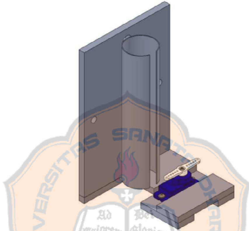
Gambar 3. 4 Servo koin
