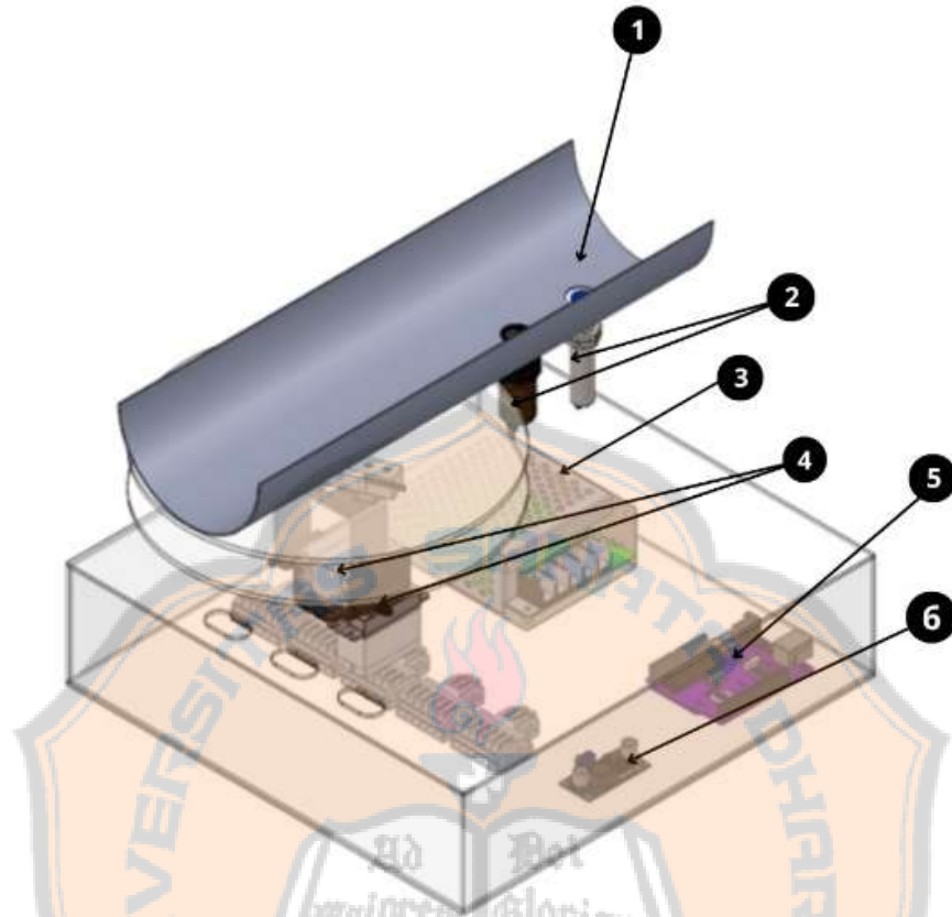
Gambar 3.3 Desain Sistem Kotak Kendali Trash2Cash
