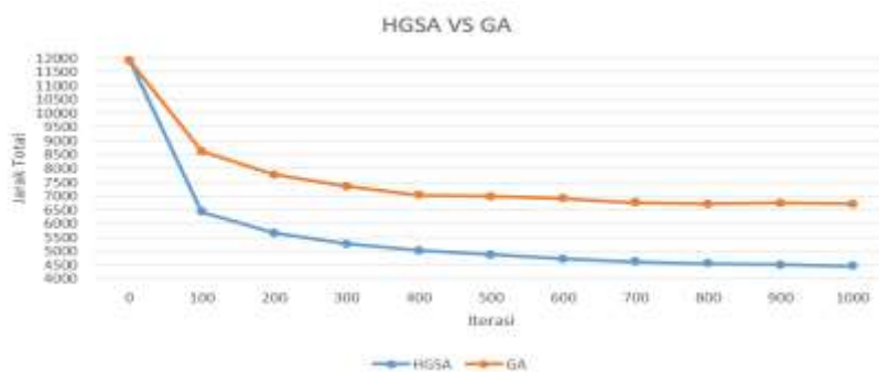
Gambar 14 Grafik HGSA vs GA
