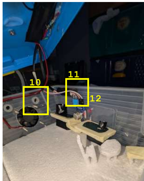
Gambar 16. Peletakan aktuator dan sensor deteksi kebakaran otomatis
